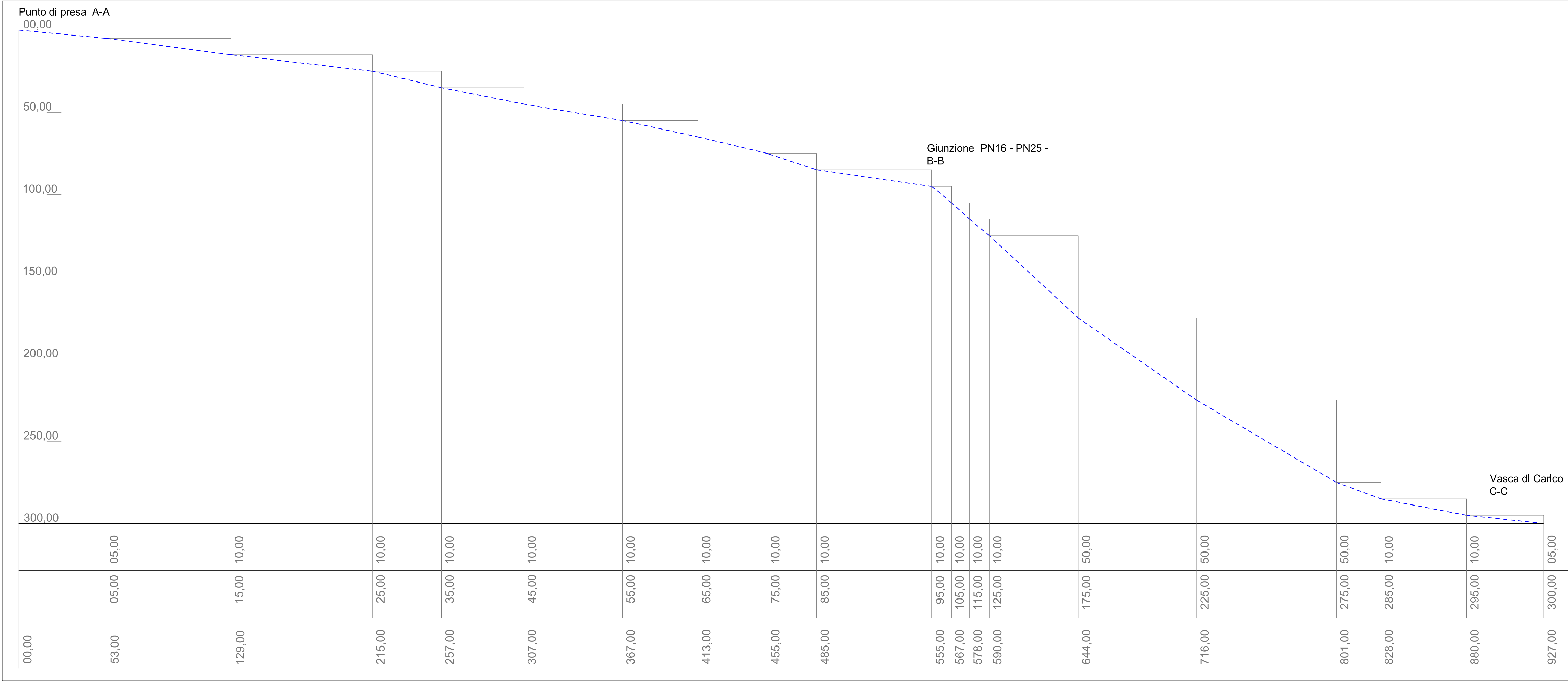
Rilievo altimetrico della condotta
